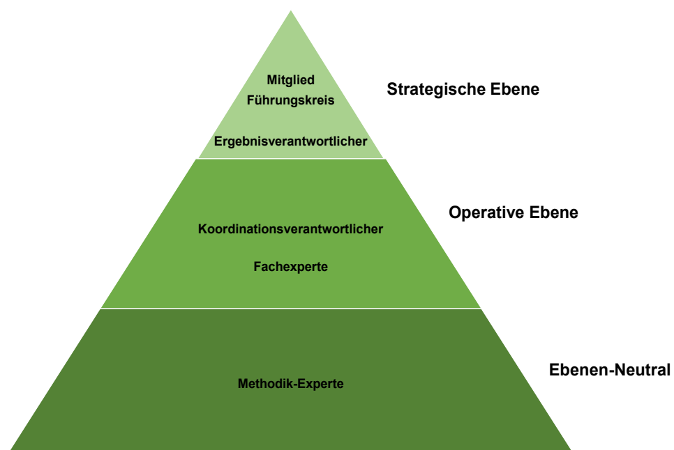
Abbildung 19 — CBPP Rollenkonzept
